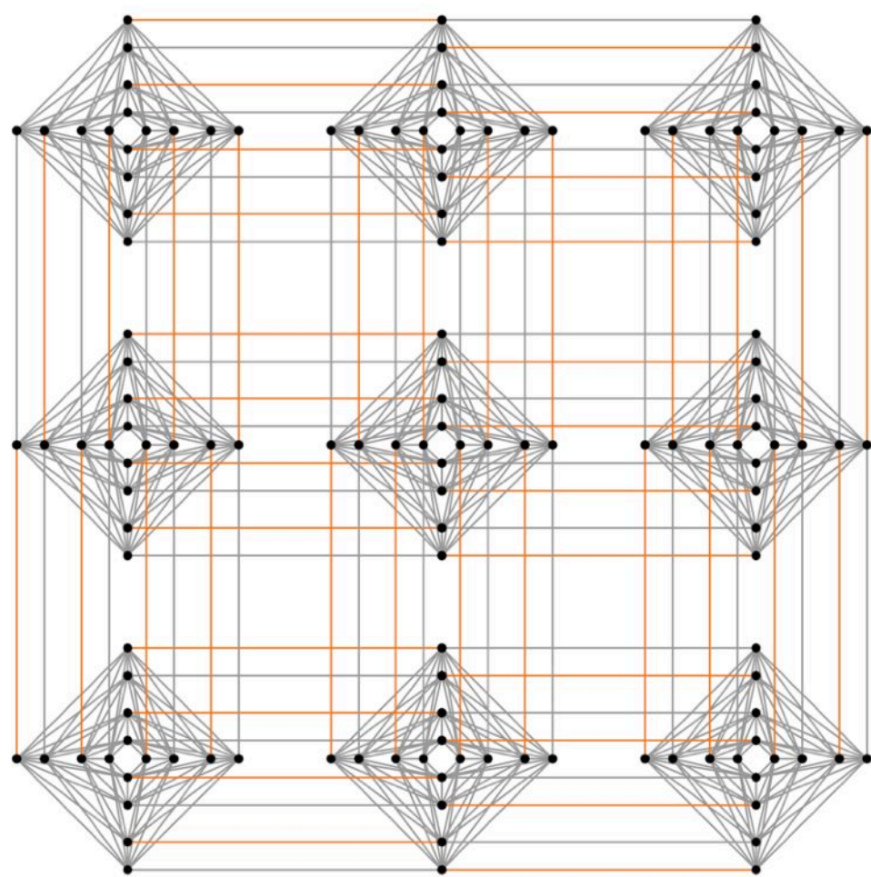
2000 Qubits
